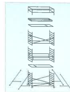
AluLight 820-C L08-00-2507-0-0 8,4 7,4 6,4
