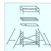
AluLight 440-C L04-00-2507-0-0 4,4 3,4 2,4
